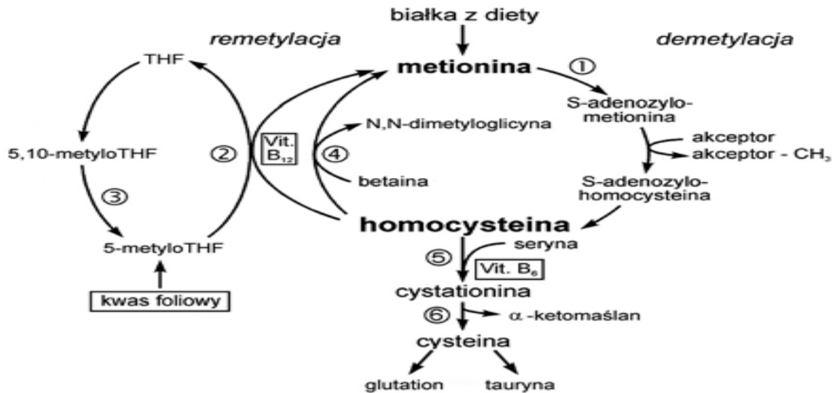
Ryc. 3 Przemiany homocysteiny[51]
